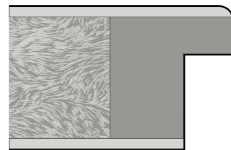
RUNDKANTE (RK) ROUNDED EDGE (RK)
