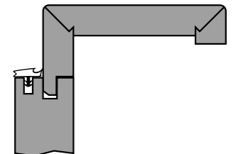
ZARGE MIT RUNDKANTE, 100 MM BEKLEIDUNG FRAME WITH ROUNDED EDGE, 100 MM CASING
