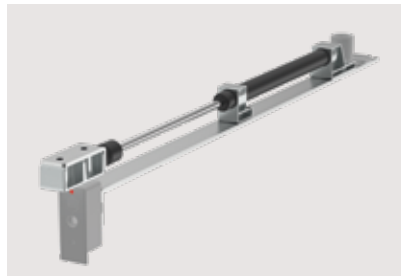
Softstop-Anschlagdämpfer
